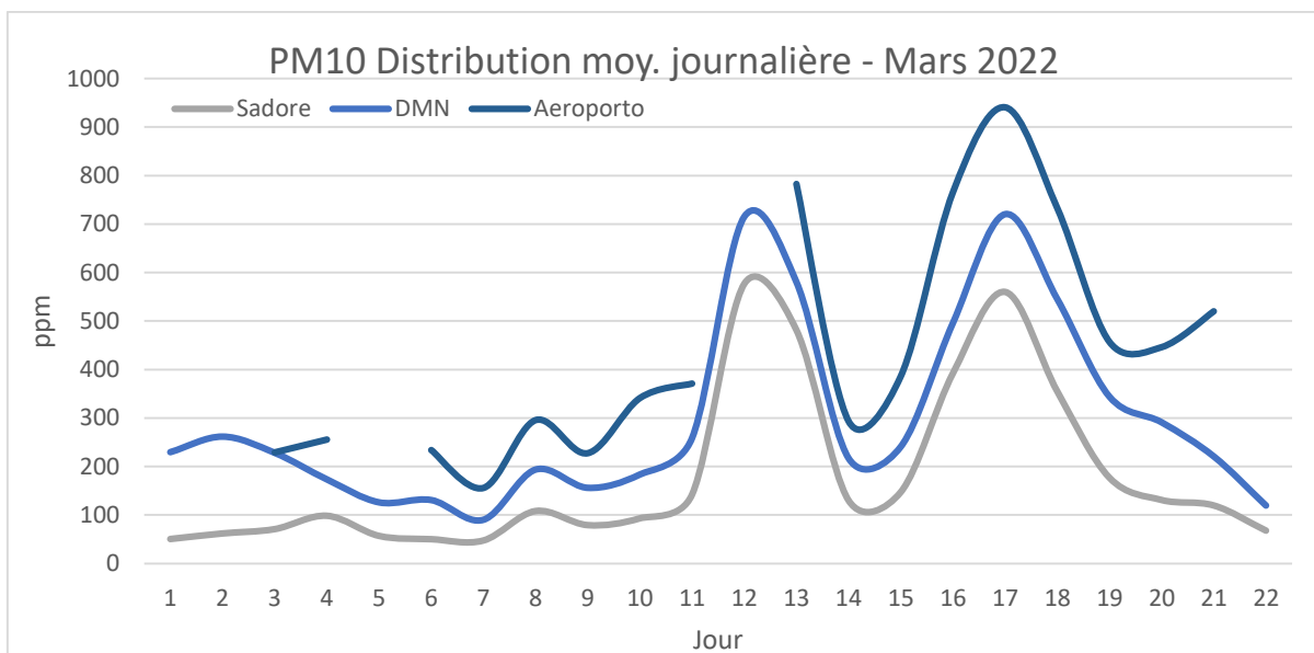
Fig. 3 Répartition journalière moyenne des PM10 à l'aéroport de Niamey, à la DMN et à Sadoré pour le mois de mars 2022
