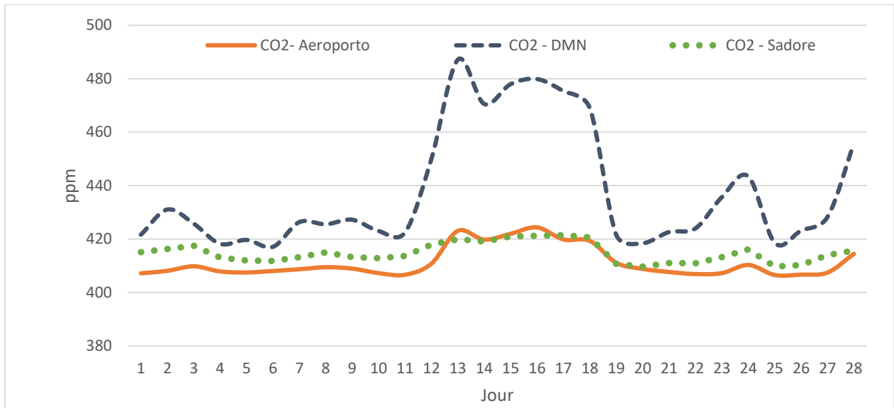
Fig. 4 Graphique de la concentration journalière moyenne de CO2 mesurée dans les stations de l'aéroport de Niamey, DMN et Sadoré en février 2022
